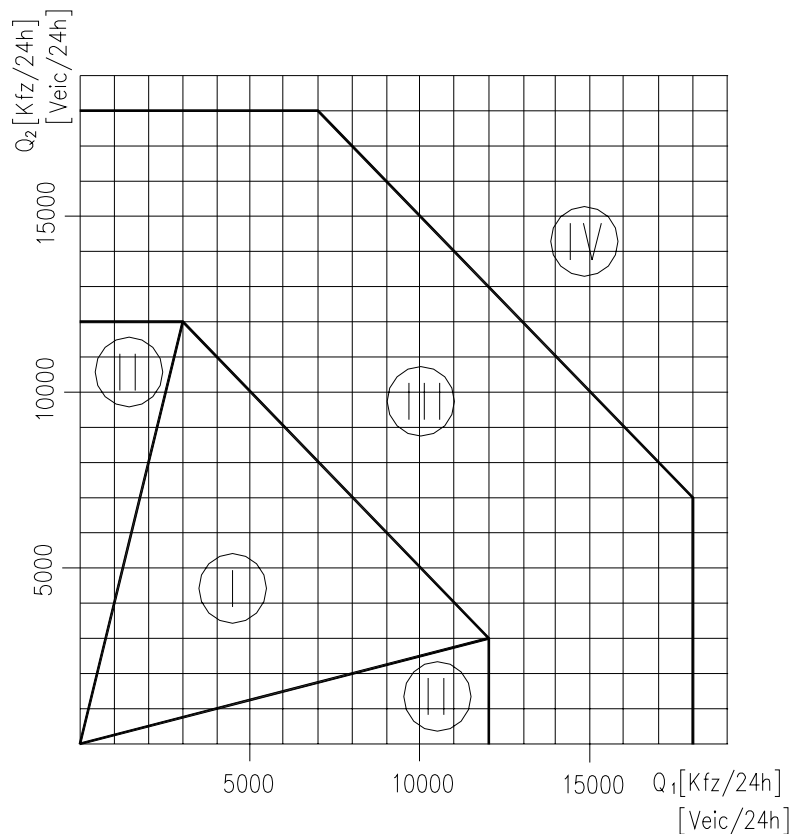
Fig. VI-05 Stima della capacità di smaltimento del traffico per una rotatoria a quattro bracci con ingressi e uscite a un'unica corsia e una corsia nella rotatoria
