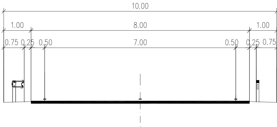
Fig. IV-03 Sezione tipo 7A
