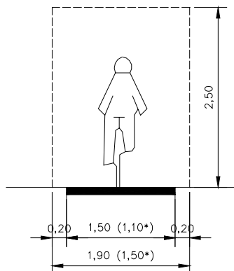
Fig. IX-01 Pista ciclabile ad una corsia con e senza la presenza di ostacoli fissi (solo lungo strade interessate da traffico motorizzato)
