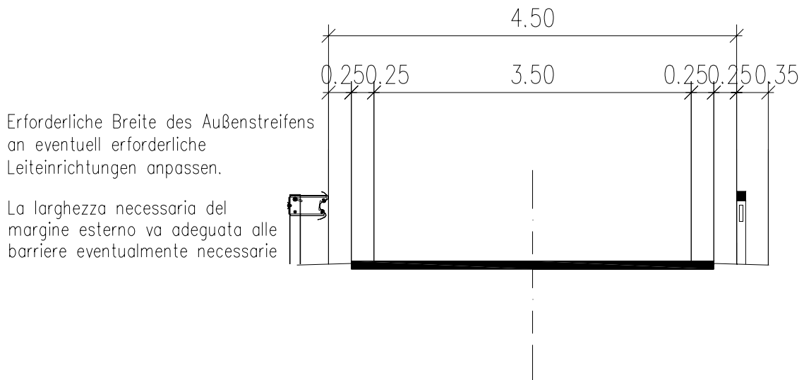
Fig. IV-08 Sezione tipo 3A
