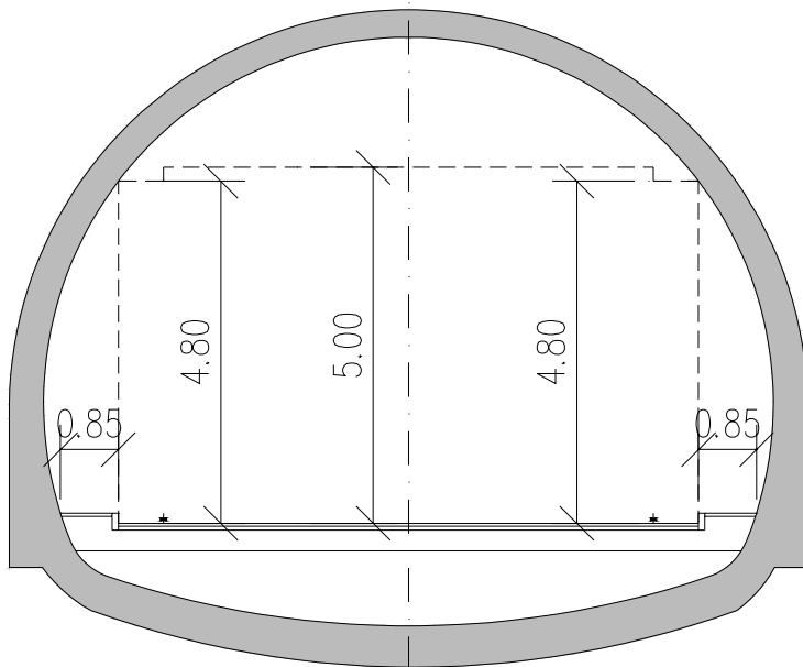
Fig. VIII-01 Sezione in galleria
