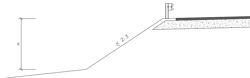
Fig. X-04 Sicurvia su scarpate
