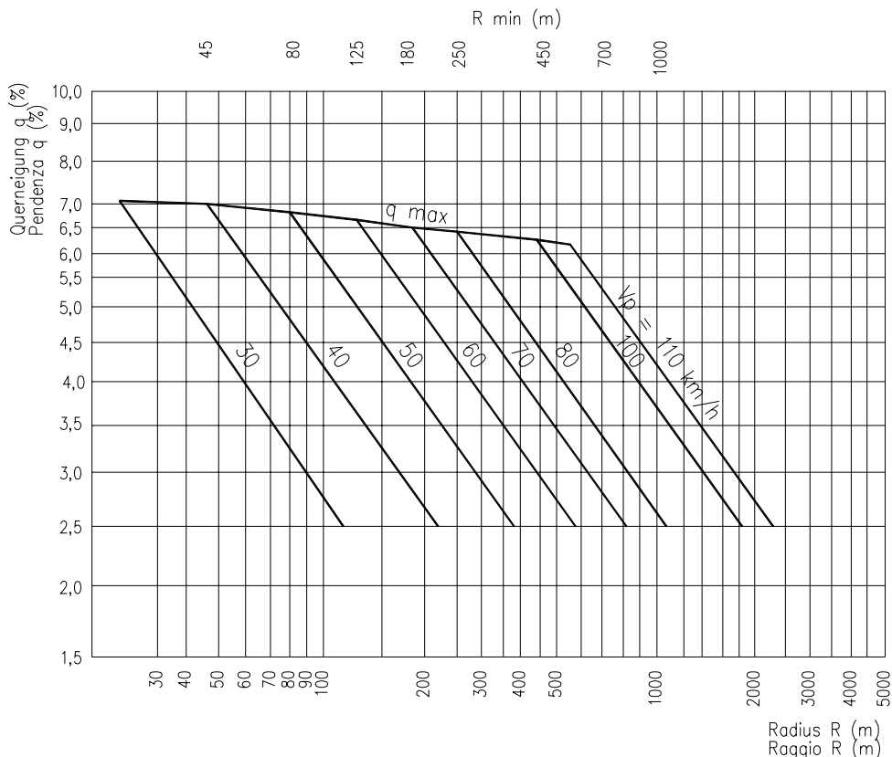
Fig. V-02 Pendenza trasversale in funzione della velocità V_p
