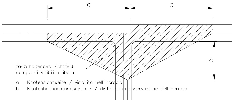
Fig. VI-04 Campo di visibilità nell'incrocio
