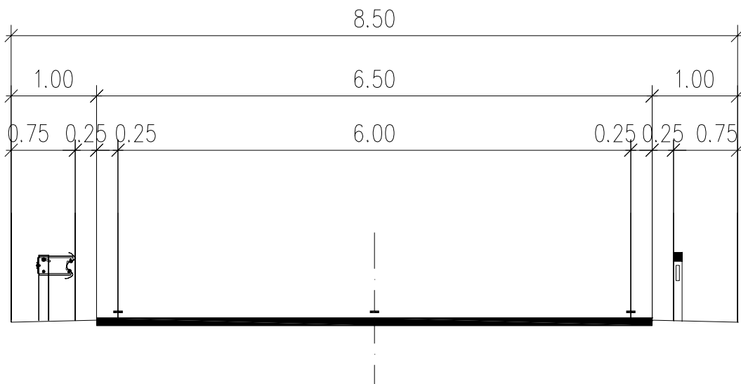
Fig. IV-06 Sezione tipo 6B
