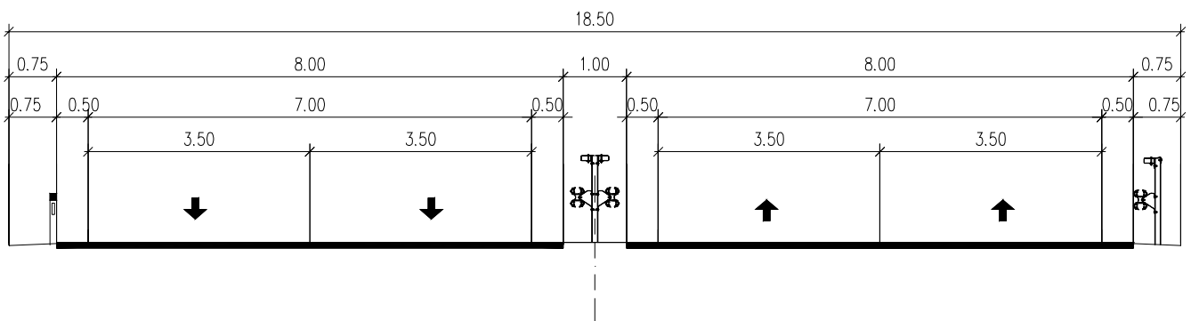
Fig. IV-02 Sezione tipo 18
