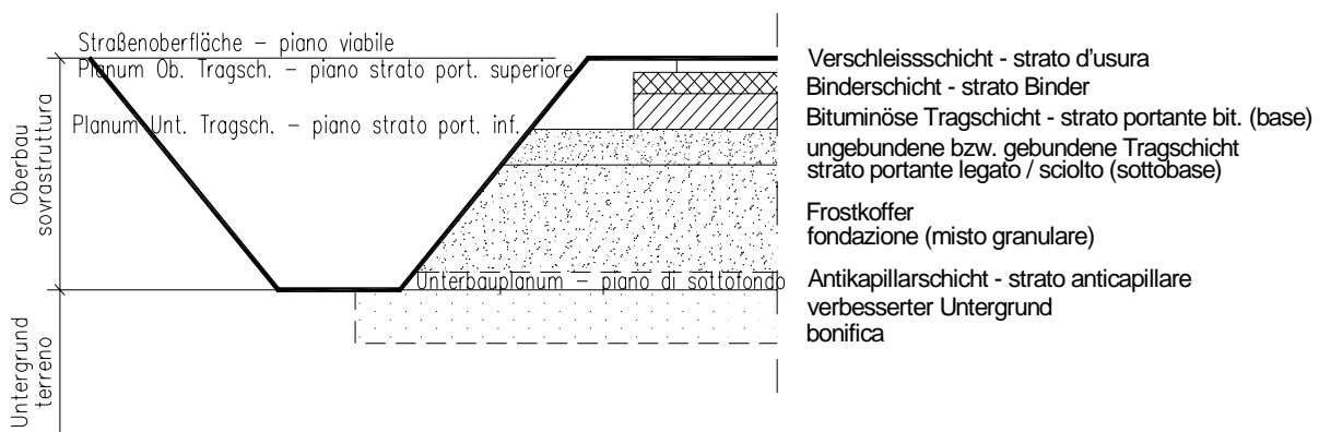
Fig. X-01 Struttura della strada (schizzo di sistema)
