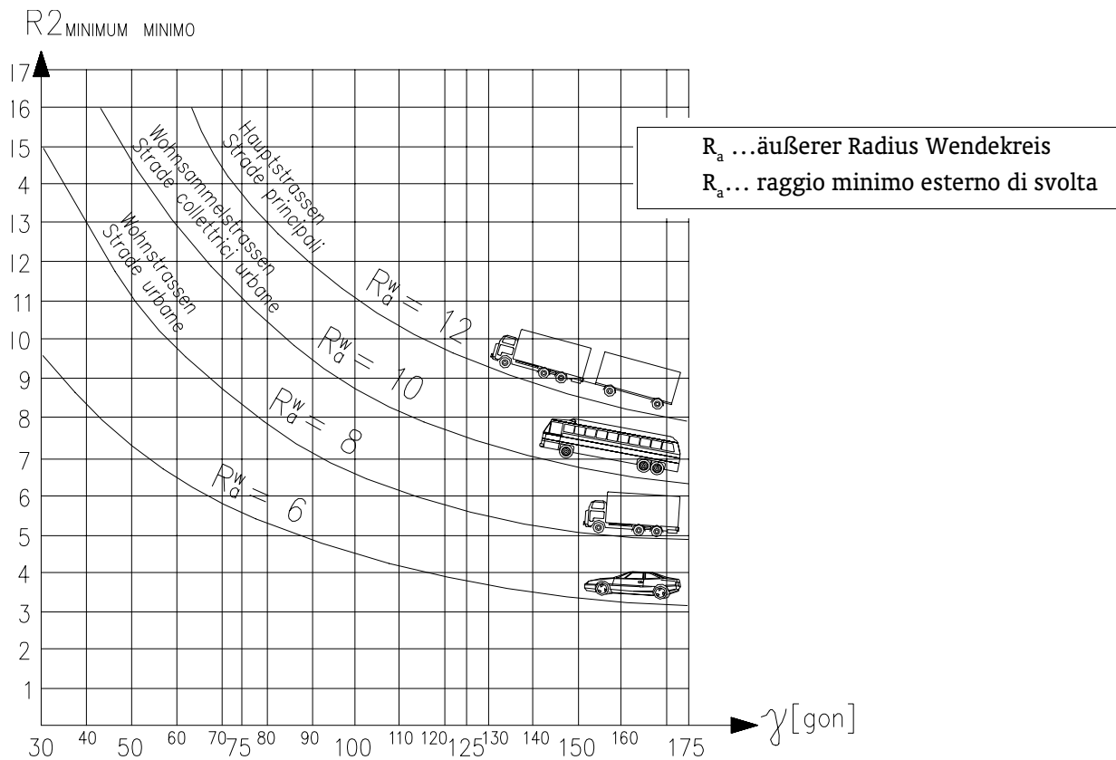
Bild VI-02 R2 abhängig vom Winkel g
