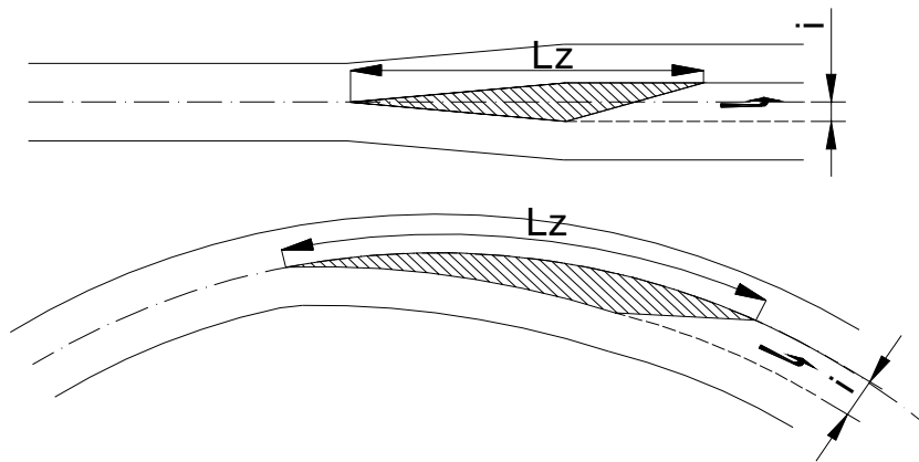
Fig. VI-03 Allargamento carreggiata i e corsia di svolta
