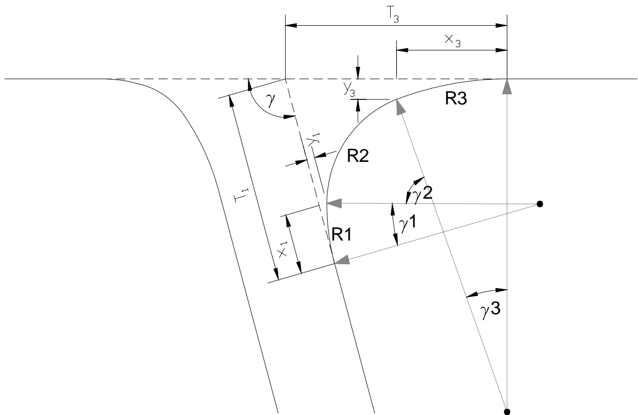
Fig. VI-01 Esecuzione di arrotondamento dell'angolo con curva tricentrica
