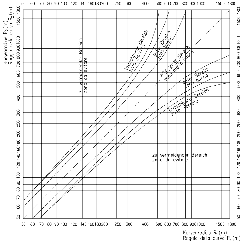
Fig. V-01 Rapporto tra i valori di due raggi di curva successivi
