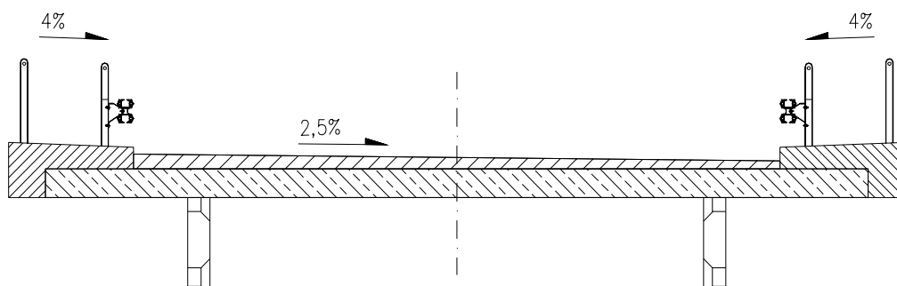
Fig. VII-01 Struttura di ponte con pendenza minima
