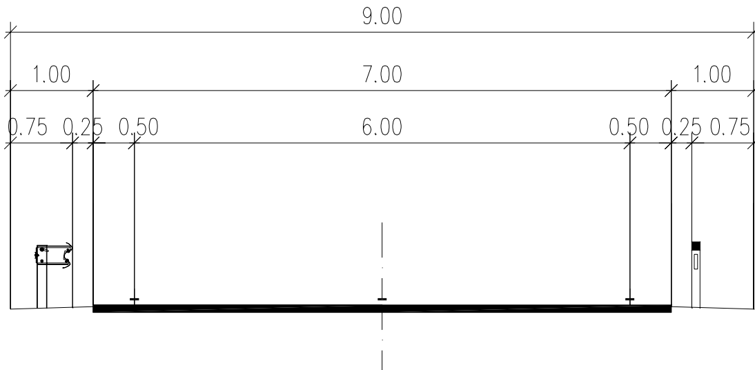
Fig. IV-05 Sezione tipo 6A
