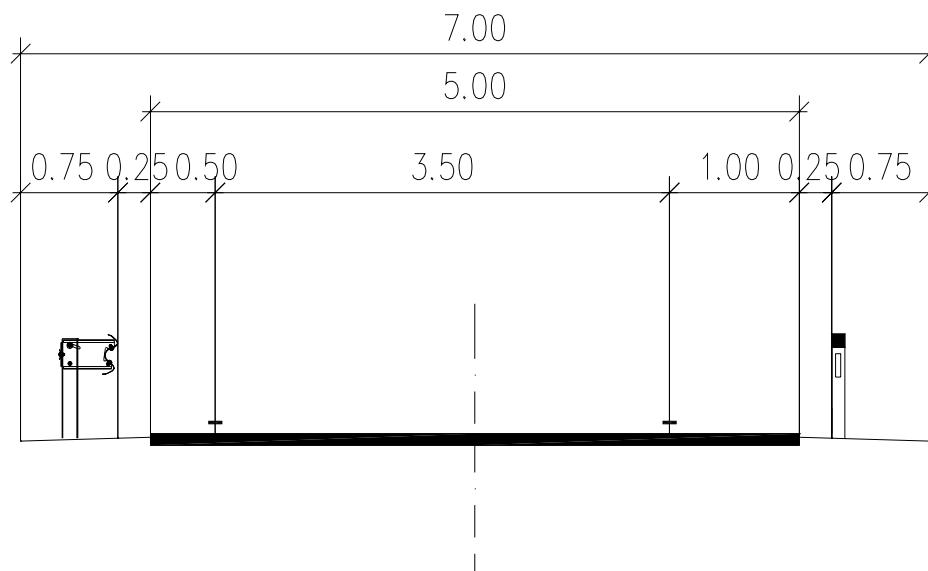
Fig. IV-10 Sezione tipo RA (rampe d'accesso)
