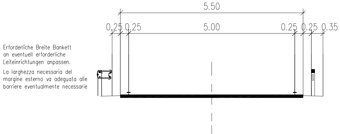
Fig. IV-07 Sezione tipo 5
