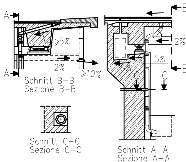
Fig. VII-02 Sistema di smaltimento acque con tubazione di scarico
