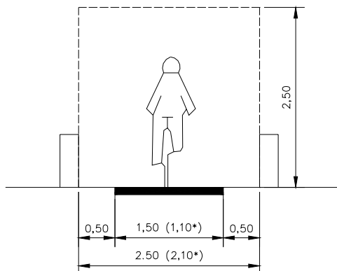
Bild IX-01 Einstreifiger Radweg mit und ohne festen Einbauten (nur längs Straßen mit motorisiertem Verkehr)
