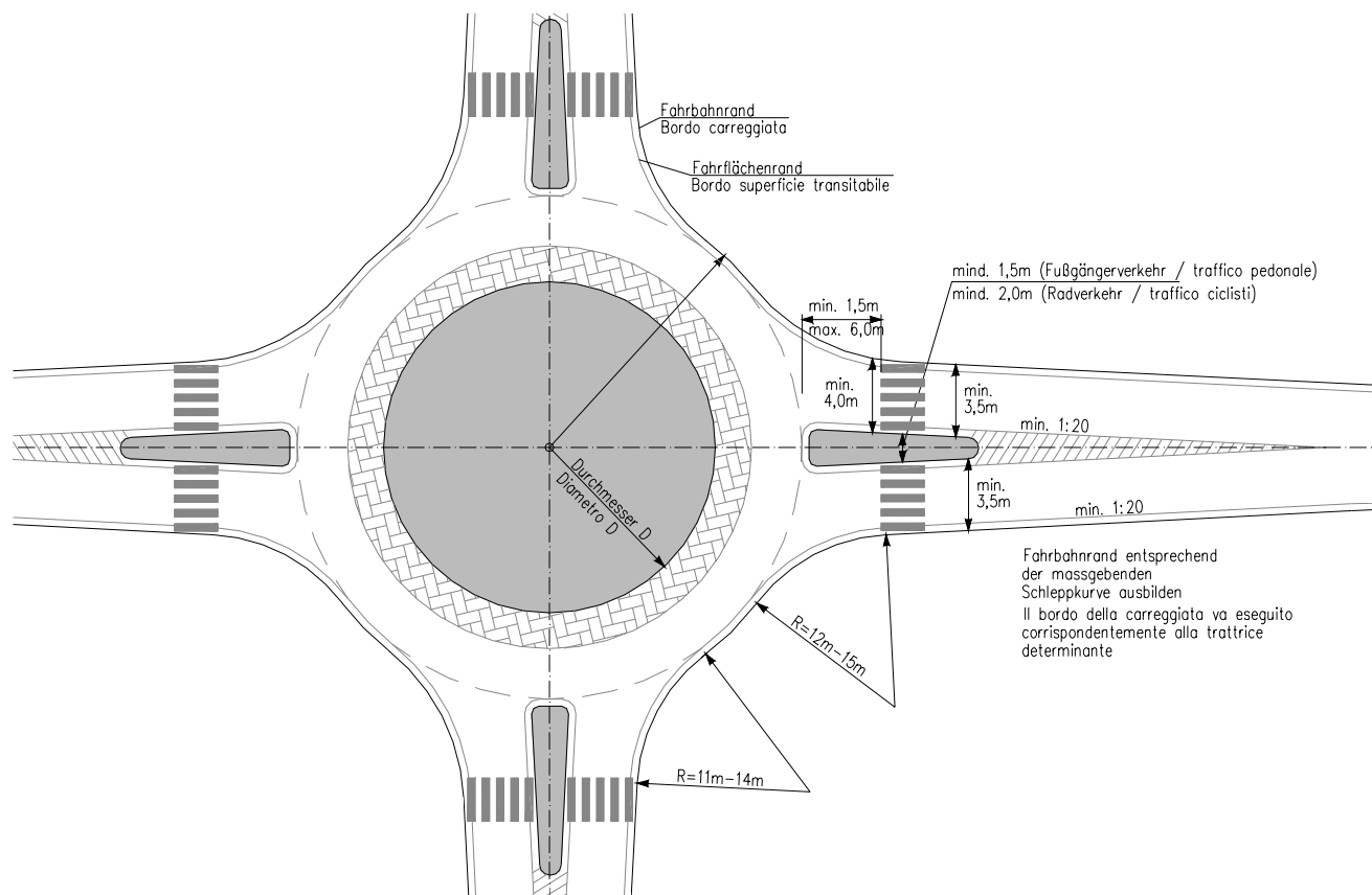
Fig. VI-07 Elementi di una piccola rotatoria
